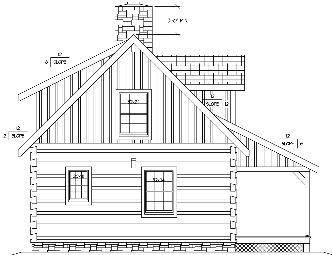
PLAN LEFT
